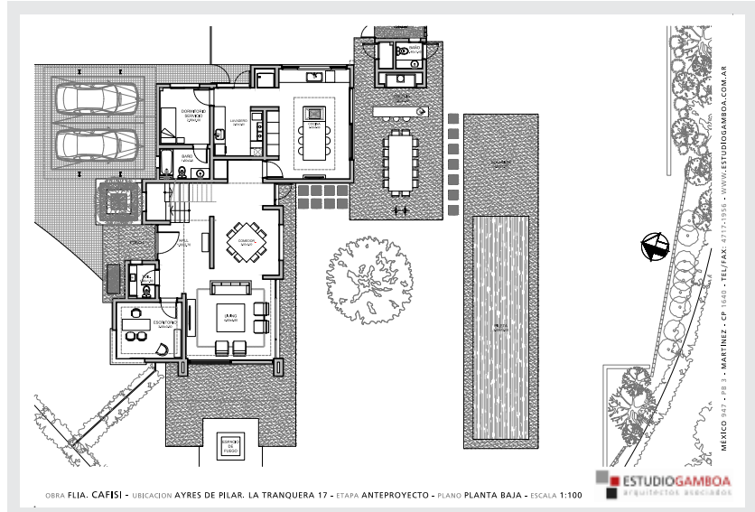
OBRA FLIA. CAFISI - UBICACION AYRES DE PILAR. LA TRANQUERA 17 - ETAPA ANTEPROYECTO - PLANO PLANTA BAJA - ESCALA 1:100
