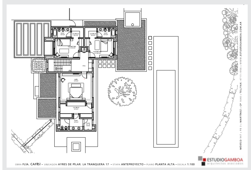
OBRA FLIA. CAFISI - UBICACION AYRES DE PILAR. LA TRANQUERA 17 - ETAPA ANTEPROYECTO - PLANO PLANTA ALTA - ESCALA 1:100
